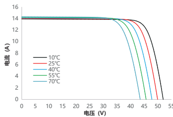
电流-电压曲线 SS8-72HS -550M
