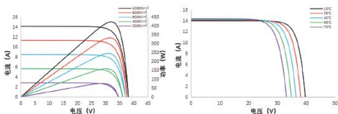
电流/功率-电压曲线 SS8-54HDT-420N
