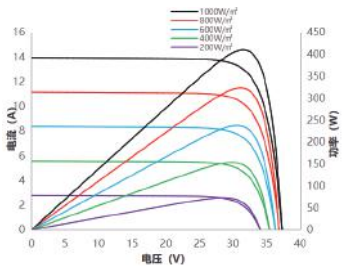
电流/功率-电压曲线 SS8-54HD -410M
