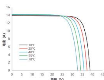
电流-电压曲线 SS8-54HD -410M
